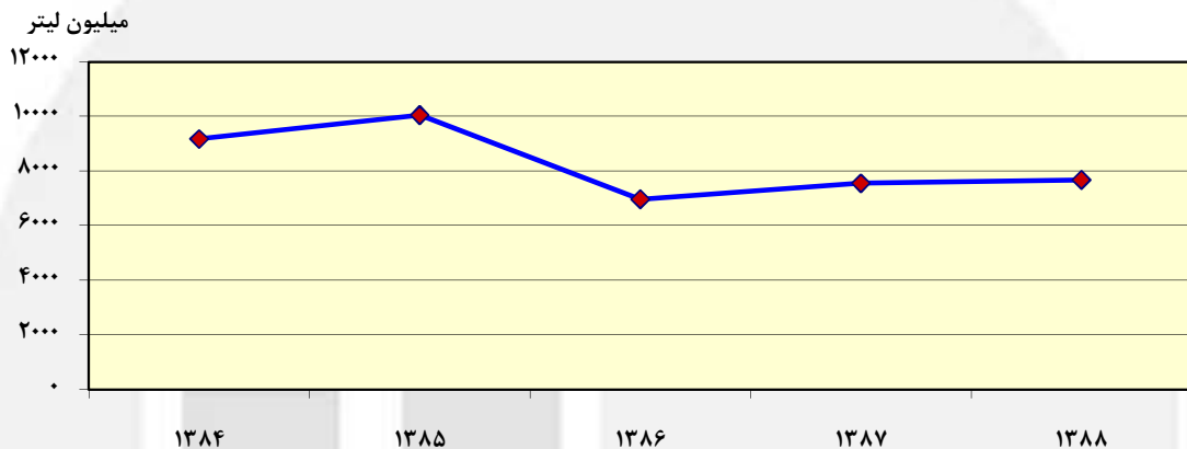
مقدار واردات بنزین موتور
