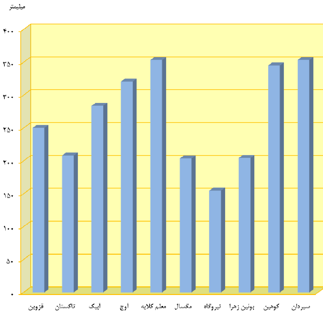
نمودار ۱-۱- بارندگی سالانه ایستگاههای هواشناسی استان: ۱۳۹۲
