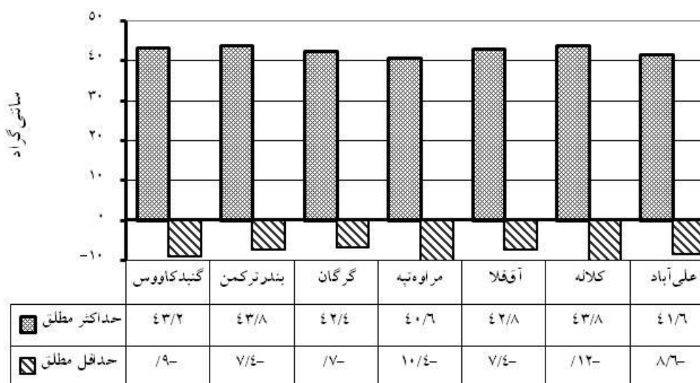
نمودار ۱-۲- حداکثر و حداقل مطلق درجهی حرارت سالانهی شهرهای استان: ۱۳۹۲
