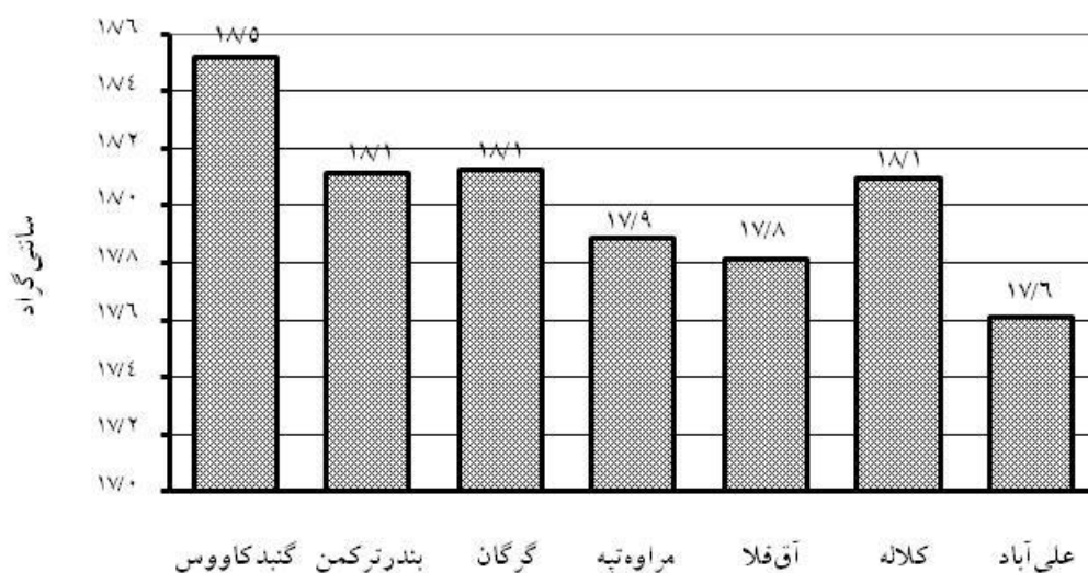
نمودار ۱-۱- متوسط درجهی حرارت سالانهی شهرهای استان: ۱۳۹۲
