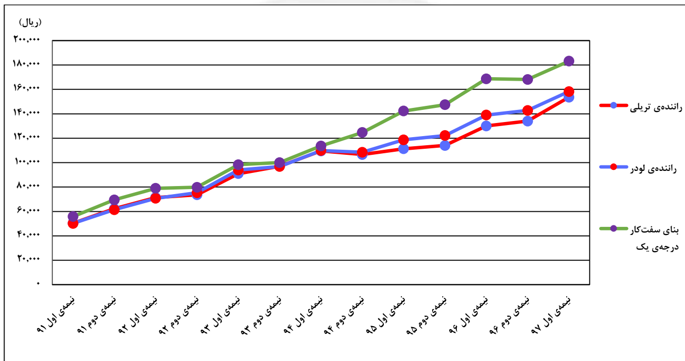
نمودار ۱- روند تغییرات متوسط دستمزد راننده‌ی تریلی، راننده‌ی لودر و بنای سفت‌کار درجه‌ی یک از نیمه‌ی اول ۱۳۹۱ تا نیمه‌ی اول ۱۳۹۷
