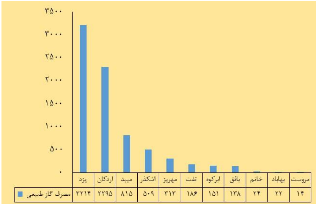
۱- ۷- مقدار مصرف گاز طبیعی استان یزد (میلیون متر مکعب)
